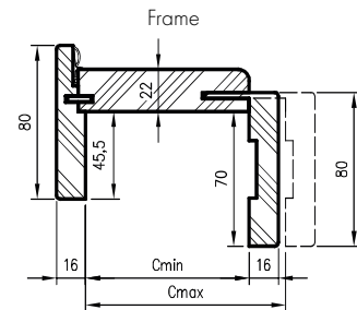
Horizontale doorsnede OF ORO
