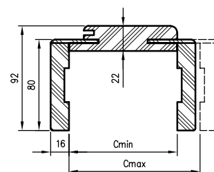
OF sectie met hoek. T80
