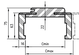
OR/ORC sectie met hoek. T63
