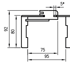
Doorsnede ORB 075
