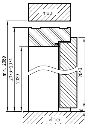
VERTICALE DOORSNEDE OP VOOR SPONNINGDEUREN
