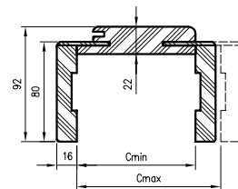
OR/ORC sectie met hoek. T80
