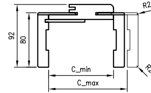
Doorsnede ORB 075
