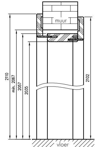
Verticale sectie van verstelbare tunnel met hoek. T63
