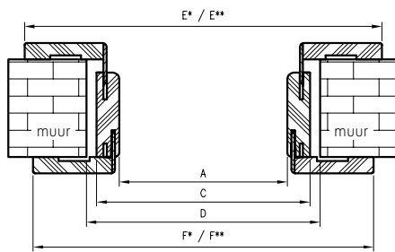
Doorsnede TUN
