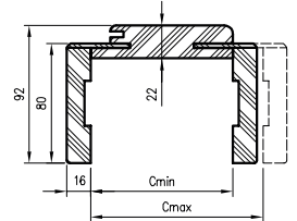
OR/ORC sectie met hoek. T80
