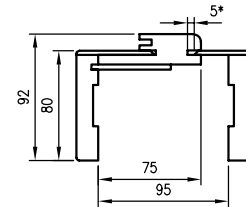
Doorsnede ORB 075
