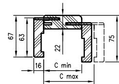
TUN sectie met hoek. T63
