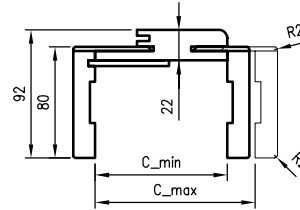
Doorsnede ORB 075
